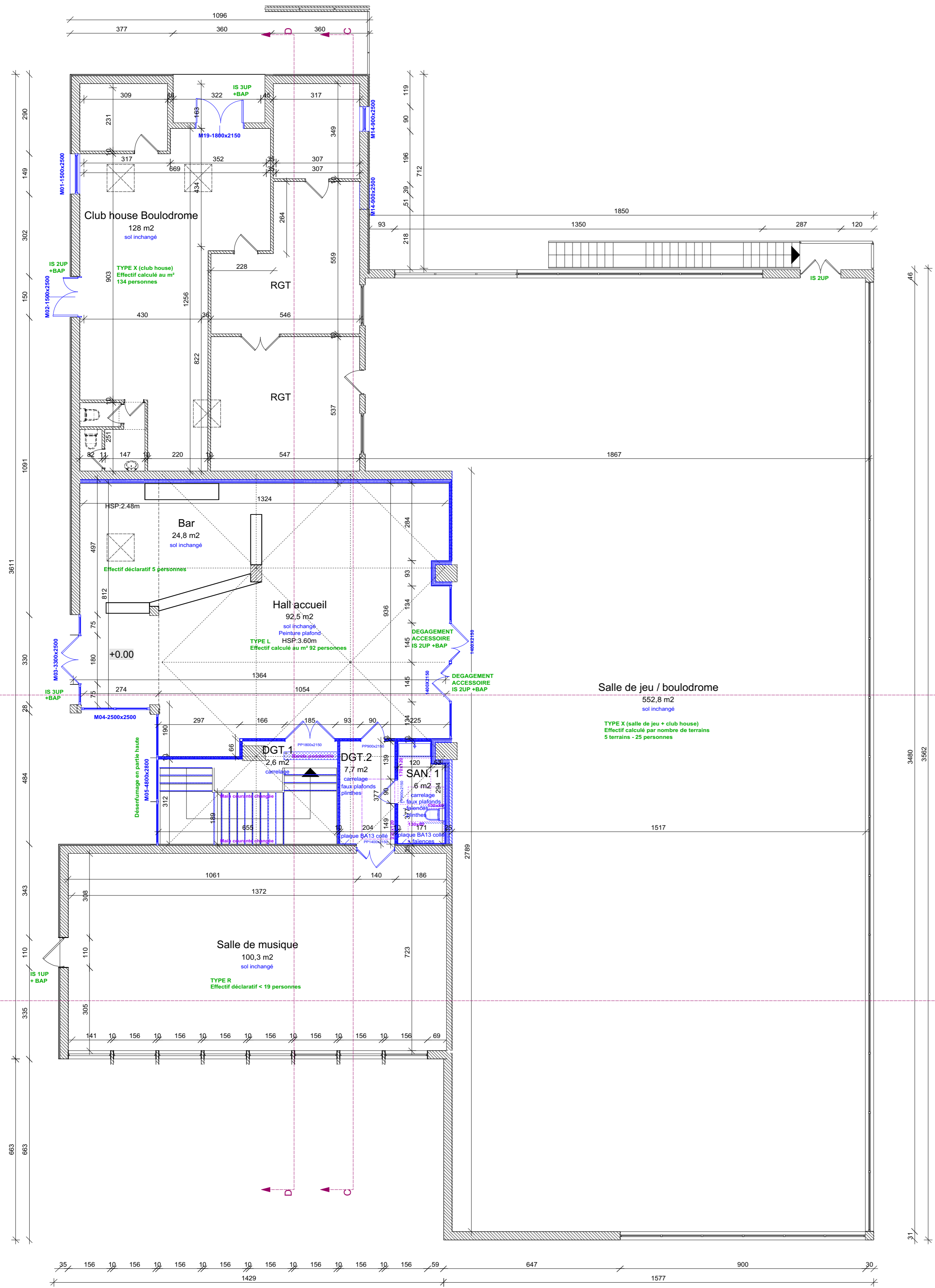
PLAN NIVEAU HAUT ECHELLE 1/100
