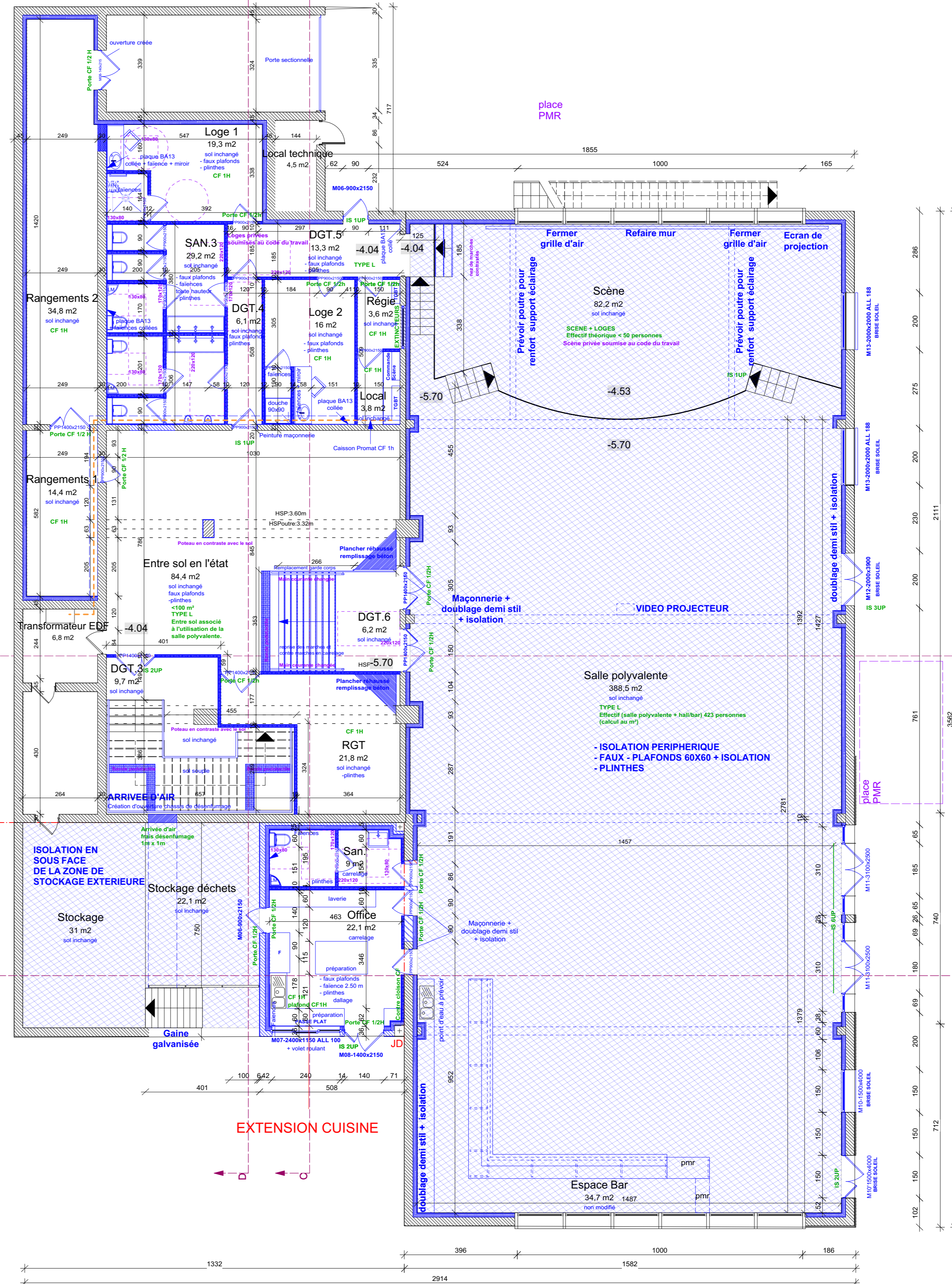
PLAN NIVEAU BAS ET ENTRE SOL 1/100
